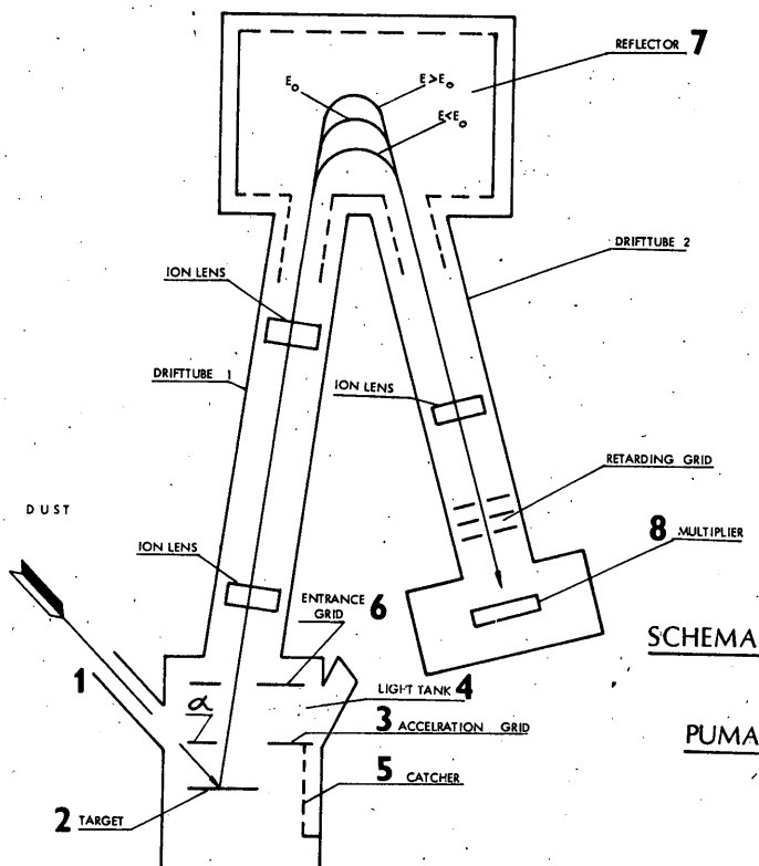
Obr. 1. Schéma hmotnostního spektrometru PUMA ze sond VEGA (legenda k číslům v textu)
