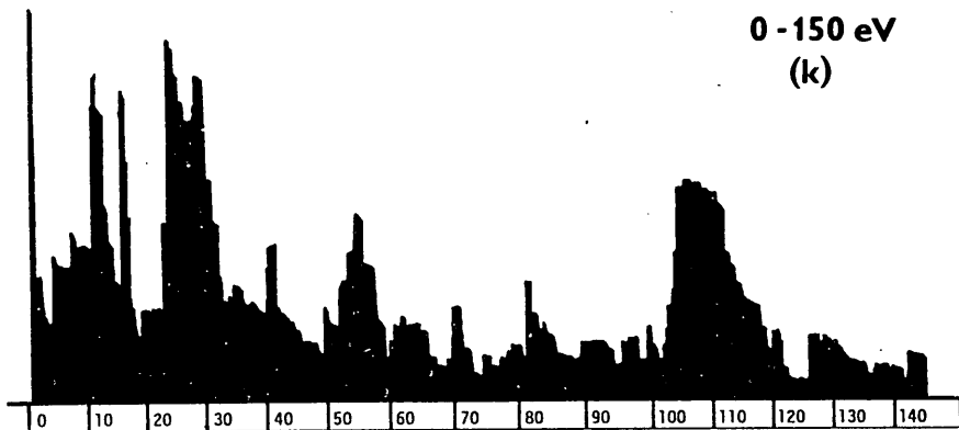
Obr. 3,4. Souborná spektra 1194 částic registrovaných spektrometrem FUMA 1 v modu 3. Liší se hlavně v citlivosti přístroje na lehké ionty H C N O, které měly patrně vyšší počáteční energie než 50 eV a nebyly proto v dostatečné míře zachyceny na tzv. dlouhých spektrech (d), zatímco na krátkých spektrech (k) jsou dobře patrné.
