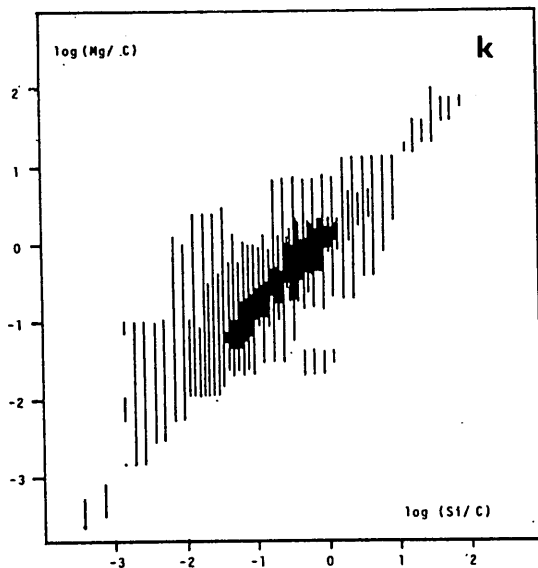
Obr. 6, 7 Korelace poměrů počtu iontů Mg/C vs. Si/C (d - dlou- há spektra, k - krátká spektra; FUMA 1 mod 3)
