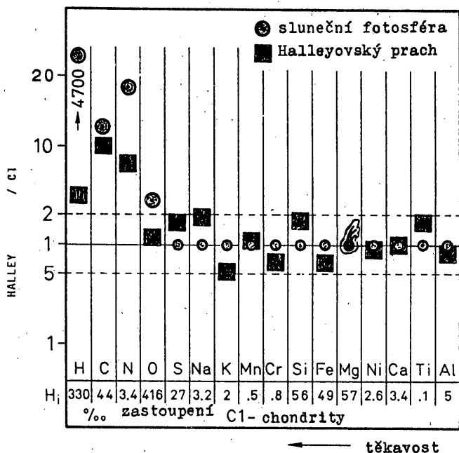
Obr. 5. Zastoupení prvků v kometárním prachu v porovnání s uhlíkatými chondrity C1 (byla použita spektra z FUMA 1 mod O)
