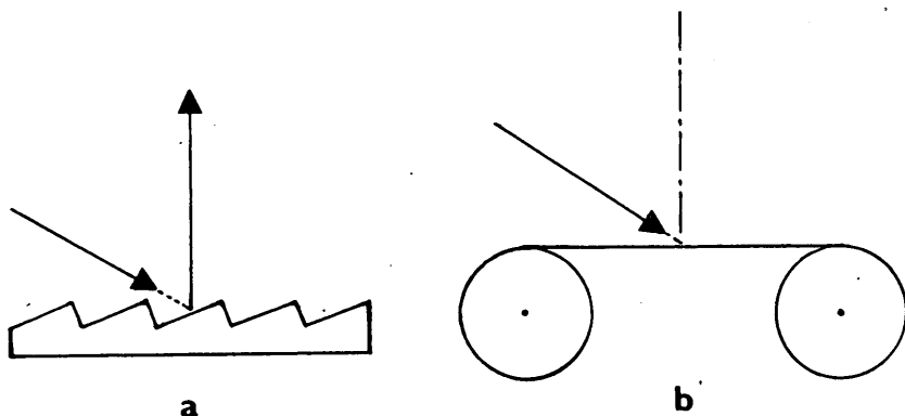
Obr. 2. Schéma terčů spektrometrů PUMA 1 (a) a PUMA 2/PIA (b). Šípka šikmo zleva označuje směr dopadu prachových zrn, směr do nitra spektrometru je kolmo vzhůru.
