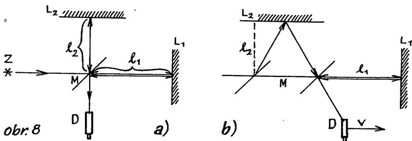
obr. 8 Schema pokusu z hlediska soustavy klidné a pohybující se vůči hypotetickému éteru.
